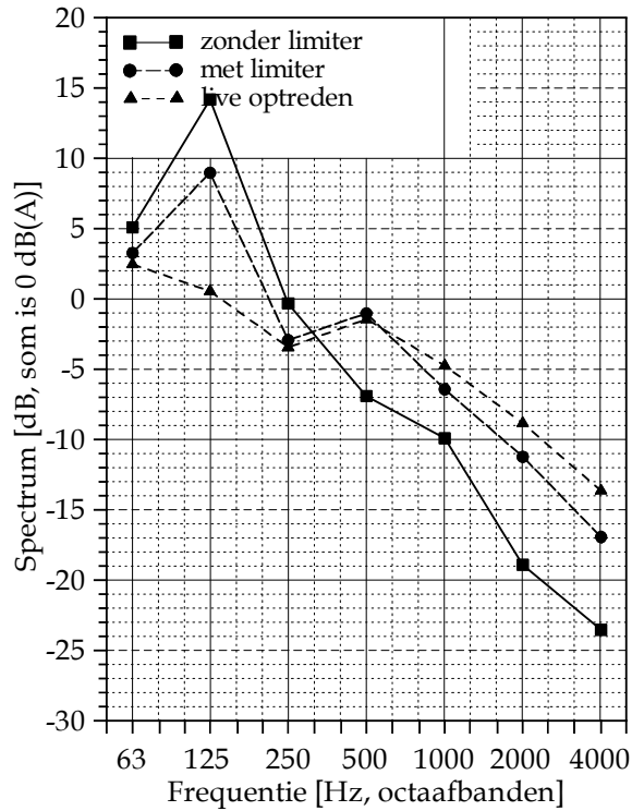
Gemeten geluidspectra in het danscafé.
