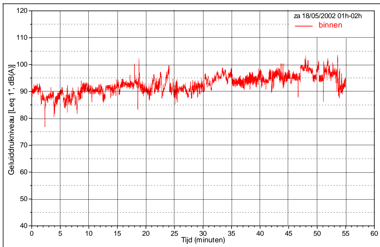
Voorbeeld van het verloop van het muziekgeluid in danscafé Kaaiman.
