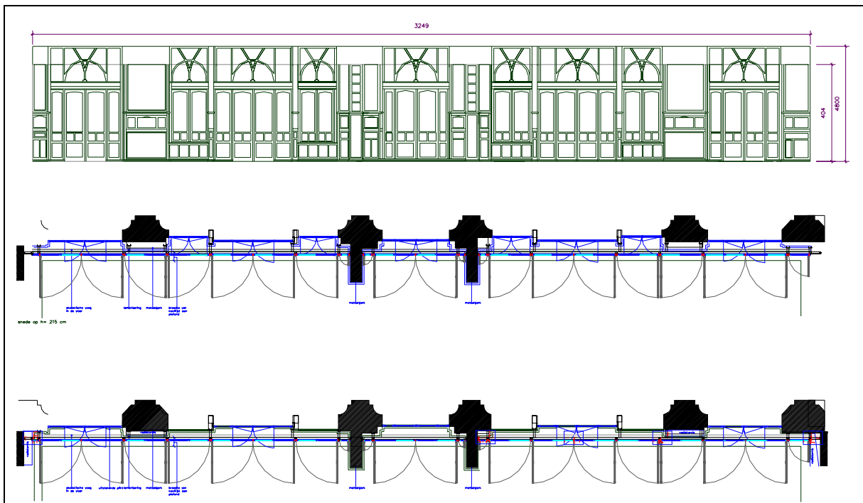
Overzichtstekening van de nieuwe voorzetramen
