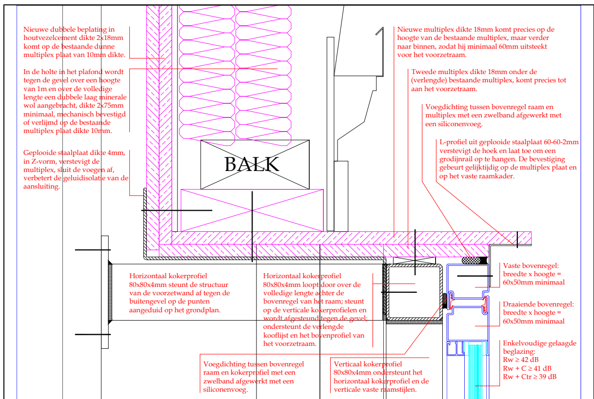
Detail van de nieuwe voorzetramen: aansluitingen in doorsnede
