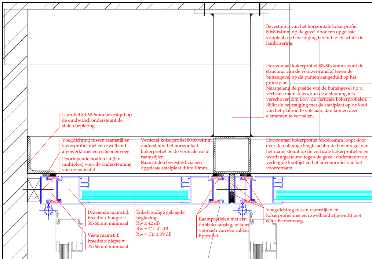
Detail van de nieuwe voorzetramen: aansluitingen in planzicht
