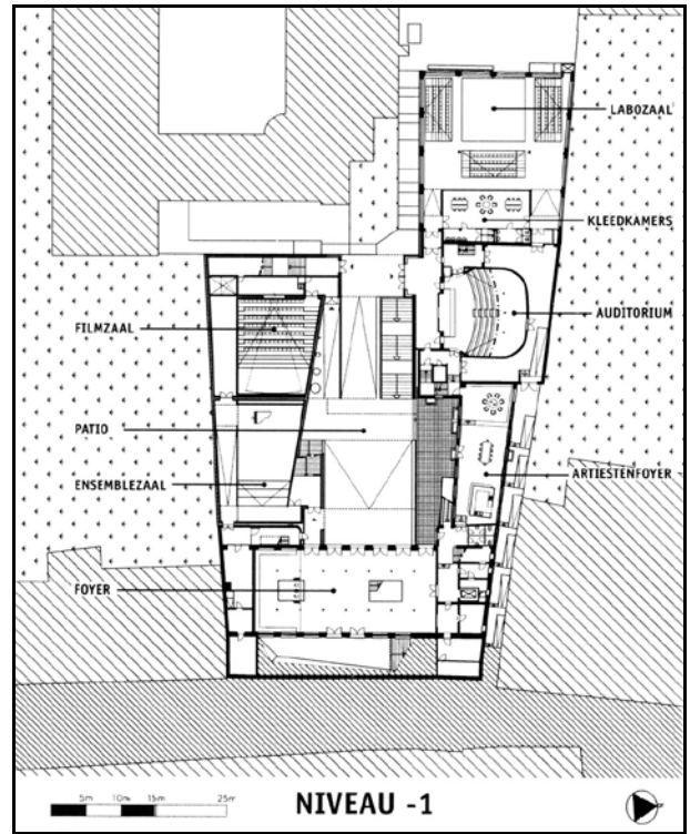
grondplan niveau -1
