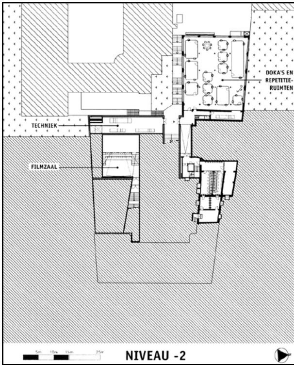
grondplan niveau -2
