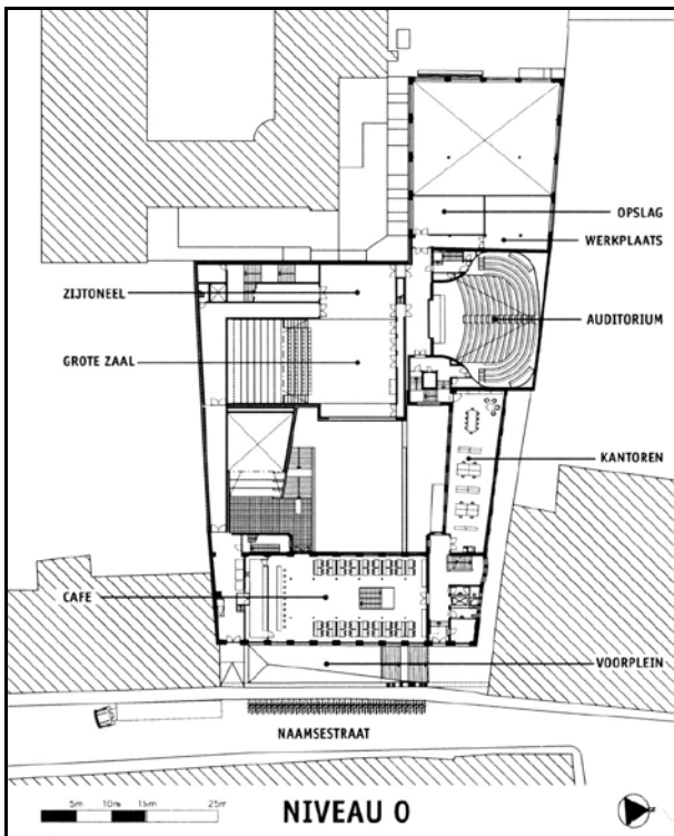
grondplan niveau 0
