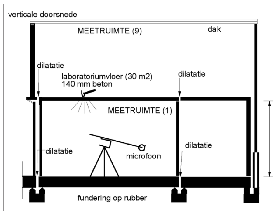
FIGUUR 1.: PEUTZ' LABORATORIUMOPSTELLING VOLGENS EN ISO 140/8
